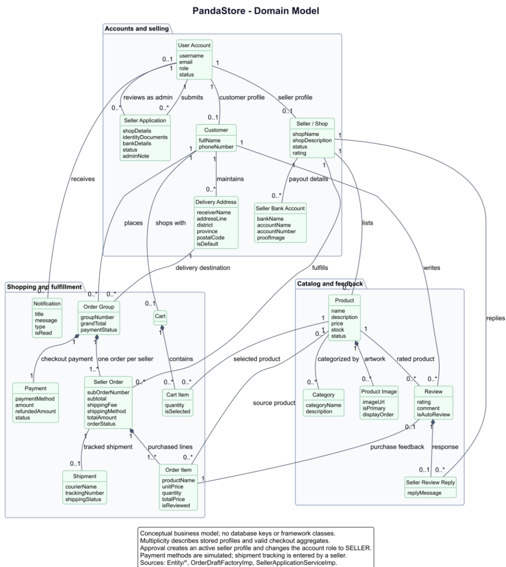
ภาพที่ 3 แบบจำลองโดเมนของ PandaStore
