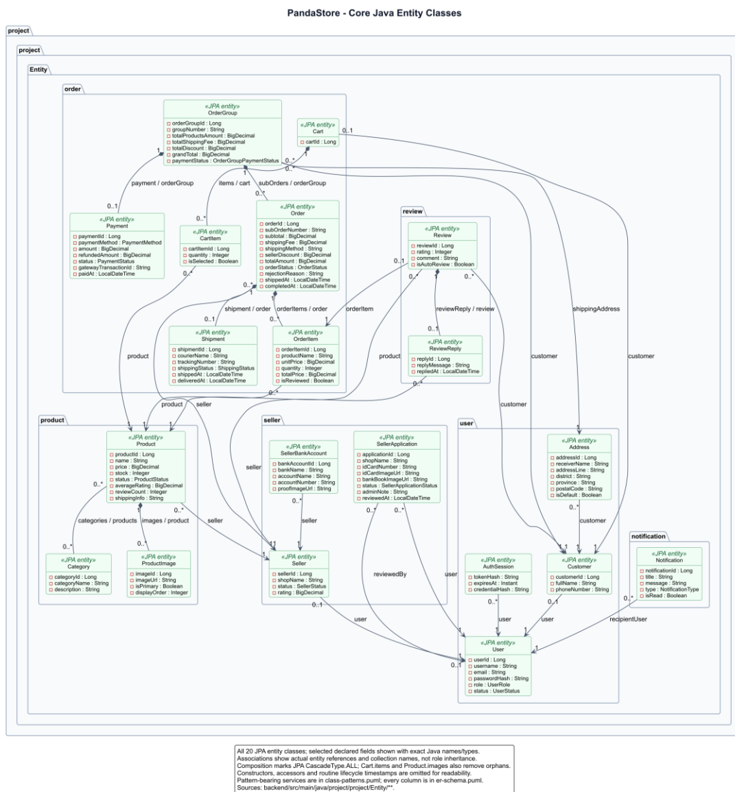
ภาพที่ 4 แผนภาพคลาสหลักของระบบ
