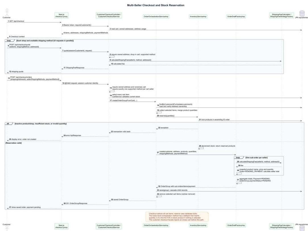
ภาพที่ 7 แผนภาพลำดับการสั่งซื้อ
