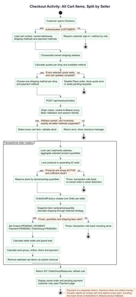
ภาพที่ 2 แผนภาพกิจกรรมการสั่งซื้อสินค้า
