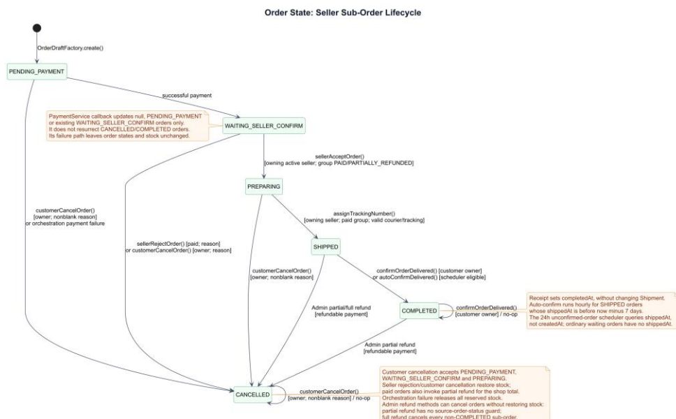
ภาพที่ 9 แผนภาพสถานะคำสั่งซื้อ
