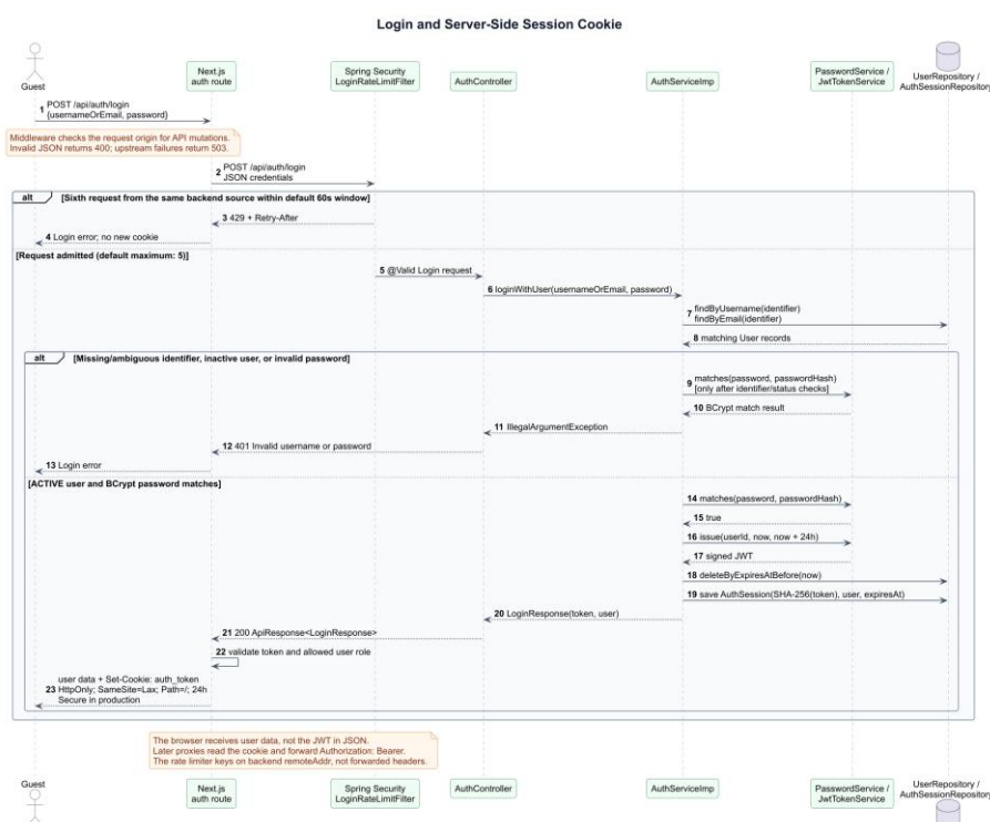
ภาพที่ 6 แผนภาพลำดับการเข้าสู่ระบบ
