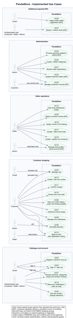
ภาพที่ 1 แผนภาพกรณีใช้งานของ PandaStore
