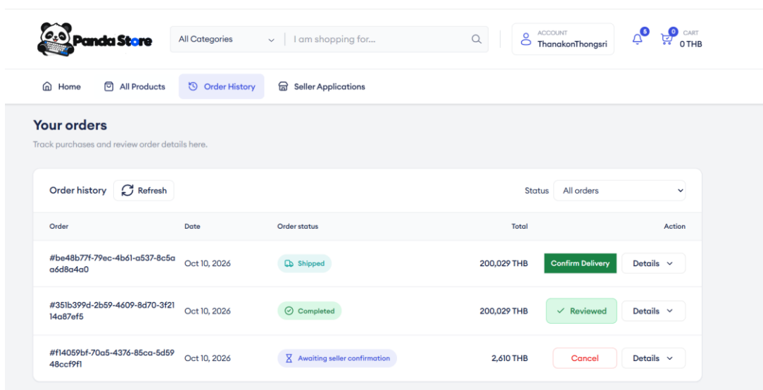
ภาพที่ 27 หน้าประวัติคำสั่งซื้อสำหรับยืนยันรับสินค้า
